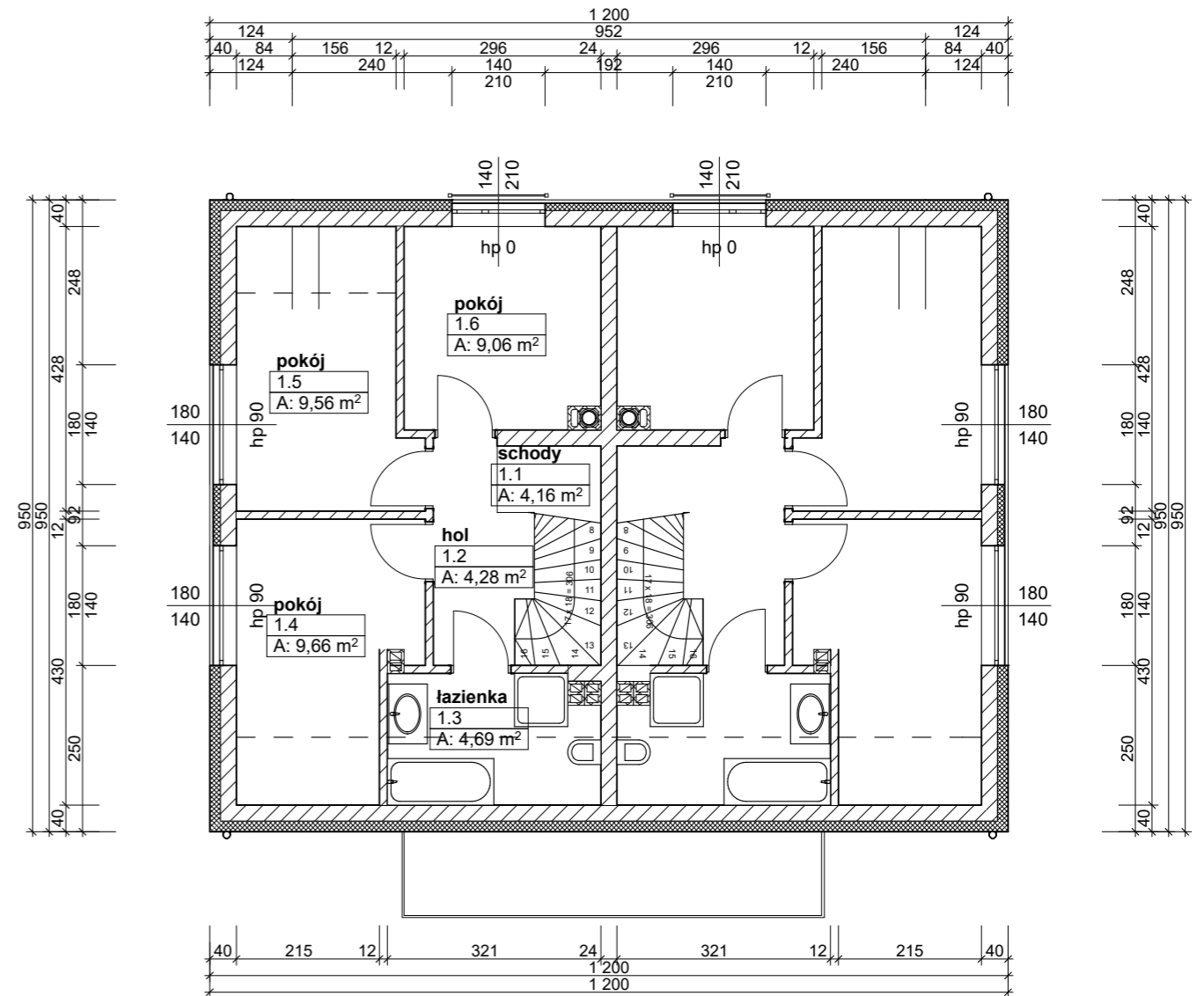
rzut pietra
