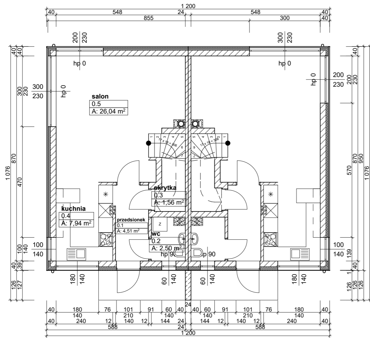
rzut parteru
